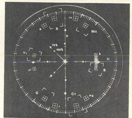
Bild 10. Vektordiagramm des Sondertestbildes
