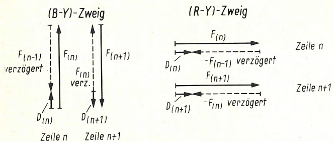
Bild 13. Zeigerdiagramm bei falscher Amplitudeneinstellung des Pal-Decoders
