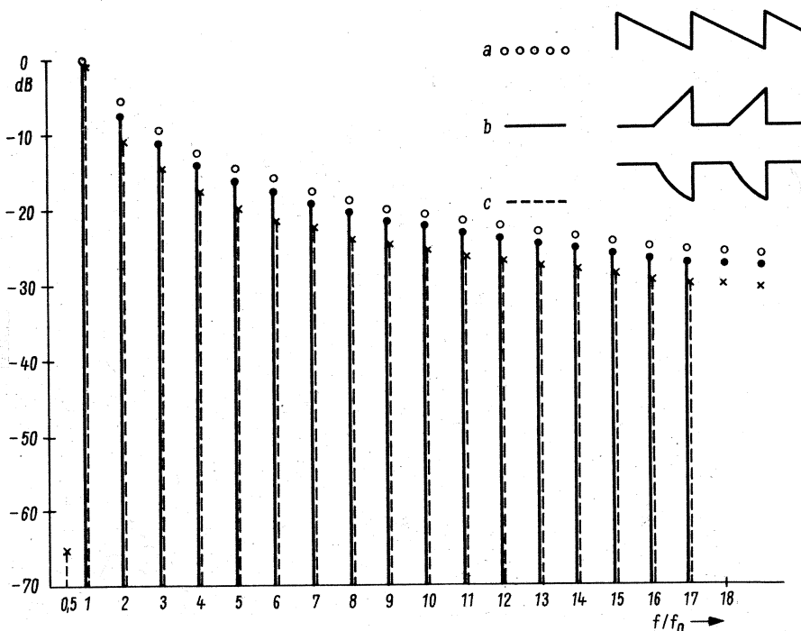
Bild 10. Frequenzspektrern verschiedener Spannungsformen bei f_0 = 1 \text{ kHz}
