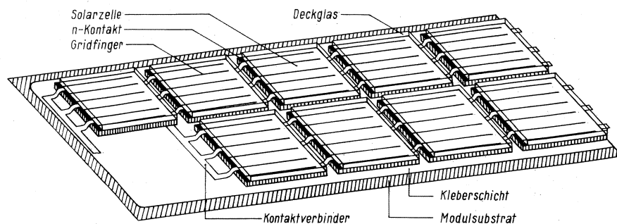
Bild 3. Schematischer Modulaufbau
