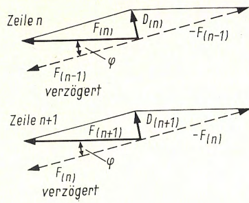
► Bild 17. Farbjalousieeffekt als Fehlerindikation des falschen Phasenabgleichs im Pal-Decoder
