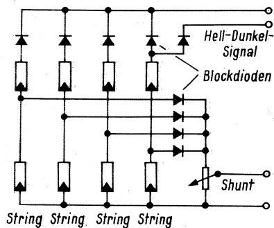
Bild 2. Blockschaltbild eines Solargenerators
