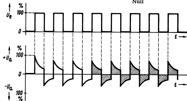
Bild 4.3. RC-Hochpaß; \tau = R \cdot C ; \tau = t_i = t_p . Einpendeln der Ausgangsspannung auf den zeitlichen Mittelwert Null
