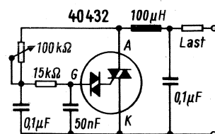
▲ Bild 1. Grundschaltung der Lichtorgel
