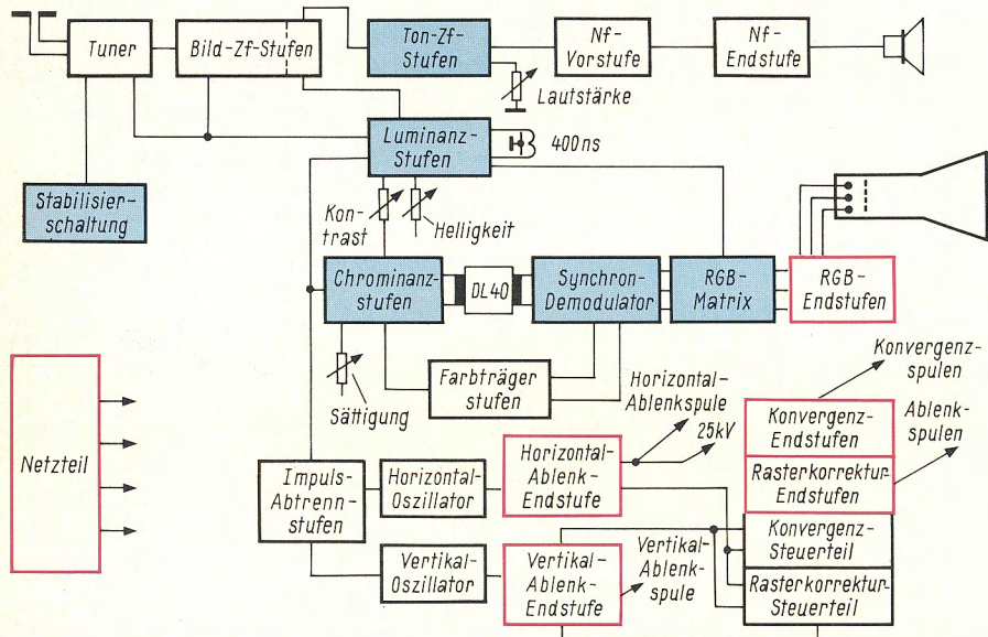
Bild 1. Blockschaltbild eines Farbfernsehempfängers. Bis auf das Netzteil und die Stufen, die unmittelbar oder mittelbar an der Bildröhre arbeiten (RGB-, Konvergenz- und Rasterkorrektur-Endstufen, Horizontal- und Vertikal-Ablenk-Endstufen, rot umrandet) lassen sich alle anderen mit integrierten Schaltungen aufbauen, obwohl einige Stufen, etwa der Tuner, z. Z. noch nicht in integrierte Form vorliegen. Die hier beschriebenen integrierten Stufen sind blau gekennzeichnet
