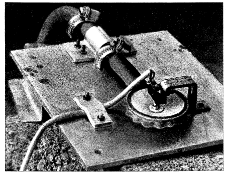
Bild 5. Der pneumatische Geber
