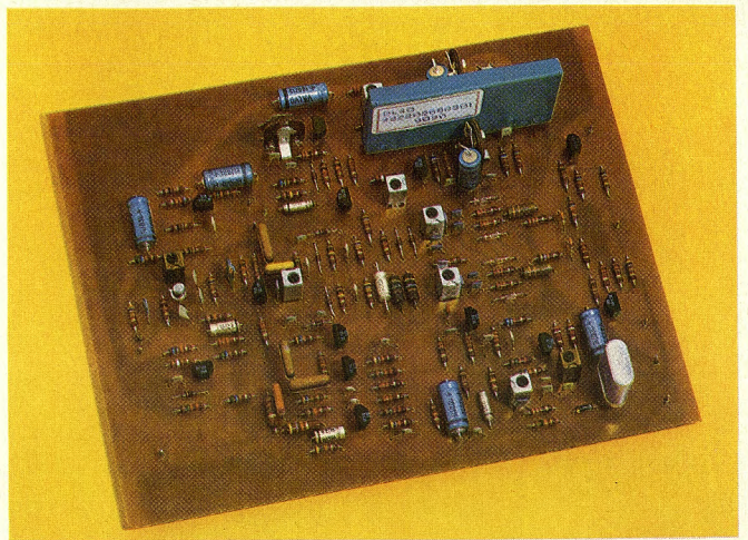
▲ Bild 2. Decoderteil mit der Einteilung in vier integrierte Schaltungen
