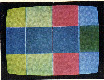
Bild 11. Sondertestbild bei verstimmtem 90°-Glied im (B-Y)-Synchrodemodulator
