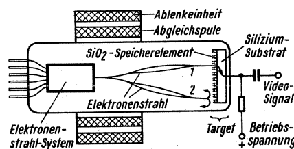
Aufbau der Silizium-Target-Speicherröhre. In dem hier gezeigten Lesebetrieb fließt bei hellen Bildstellen ein entsprechender Strom über das Siliziumsubstrat (1), während beim Schwarzwert alle Elektronen des Abtaststrahls abgestoßen werden (2).
