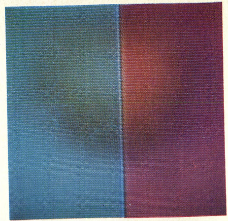
► Bild 17. Farbjalousieeffekt als Fehlerindikation des falschen Phasenabgleichs im Pal-Decoder
