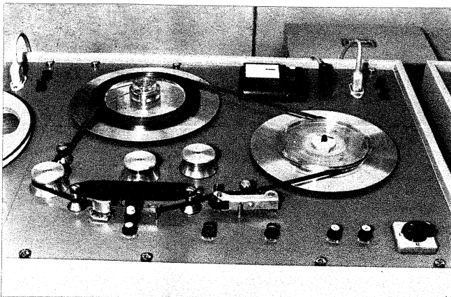
▲ Bild 3. Teilbild einer Konfektioniermaschine zum Einspulen in Kassetten
