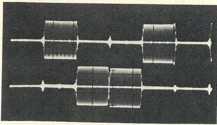
Bild 5. Geträgertes (R - Y)- und (B - Y)-Signal bei richtig abgeglichenem Pal-Decoder
